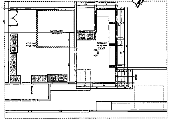
DET. 2 PLANTA DEMOLIR E CONSTRUIR ESC. 1/75
